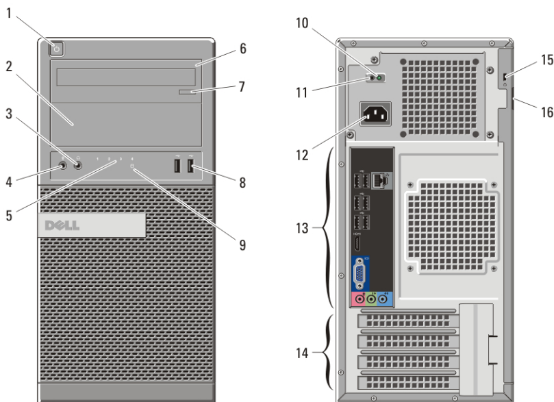
Figura 1. Vista anteriore e posteriore Minitorre
